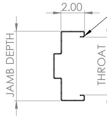
JAMB & HEADER PROFILE
